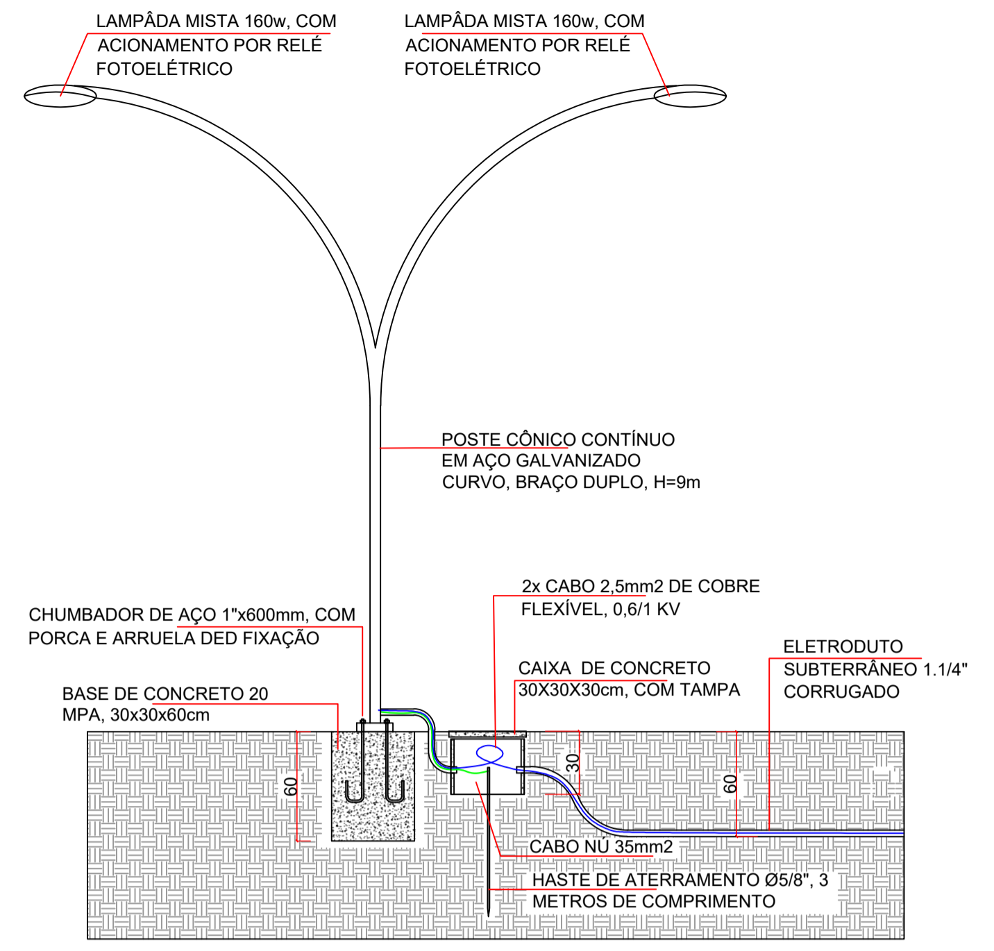
DETALHE INSTALAÇÃO POSTE CÔNICO
