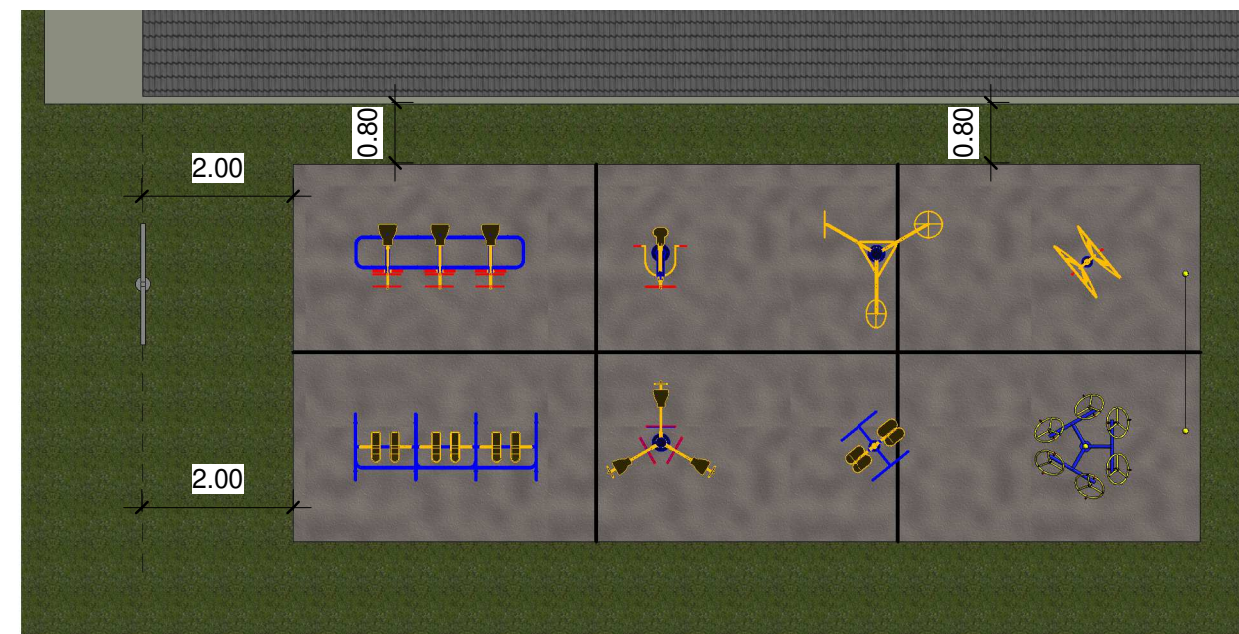
3 BS - Localização Detalhe 1 : 100
