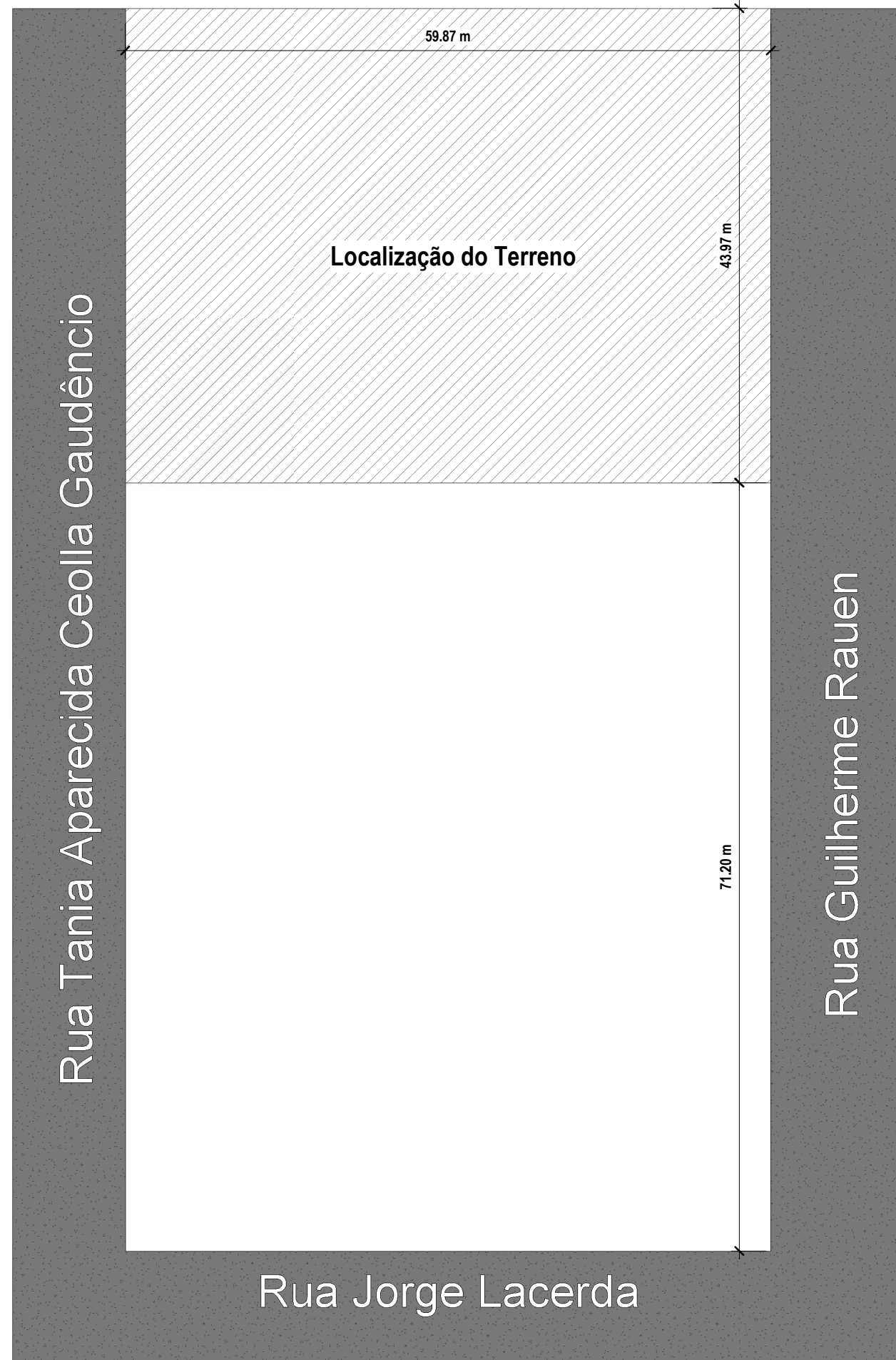
1 Planta de Situação 1 : 500
