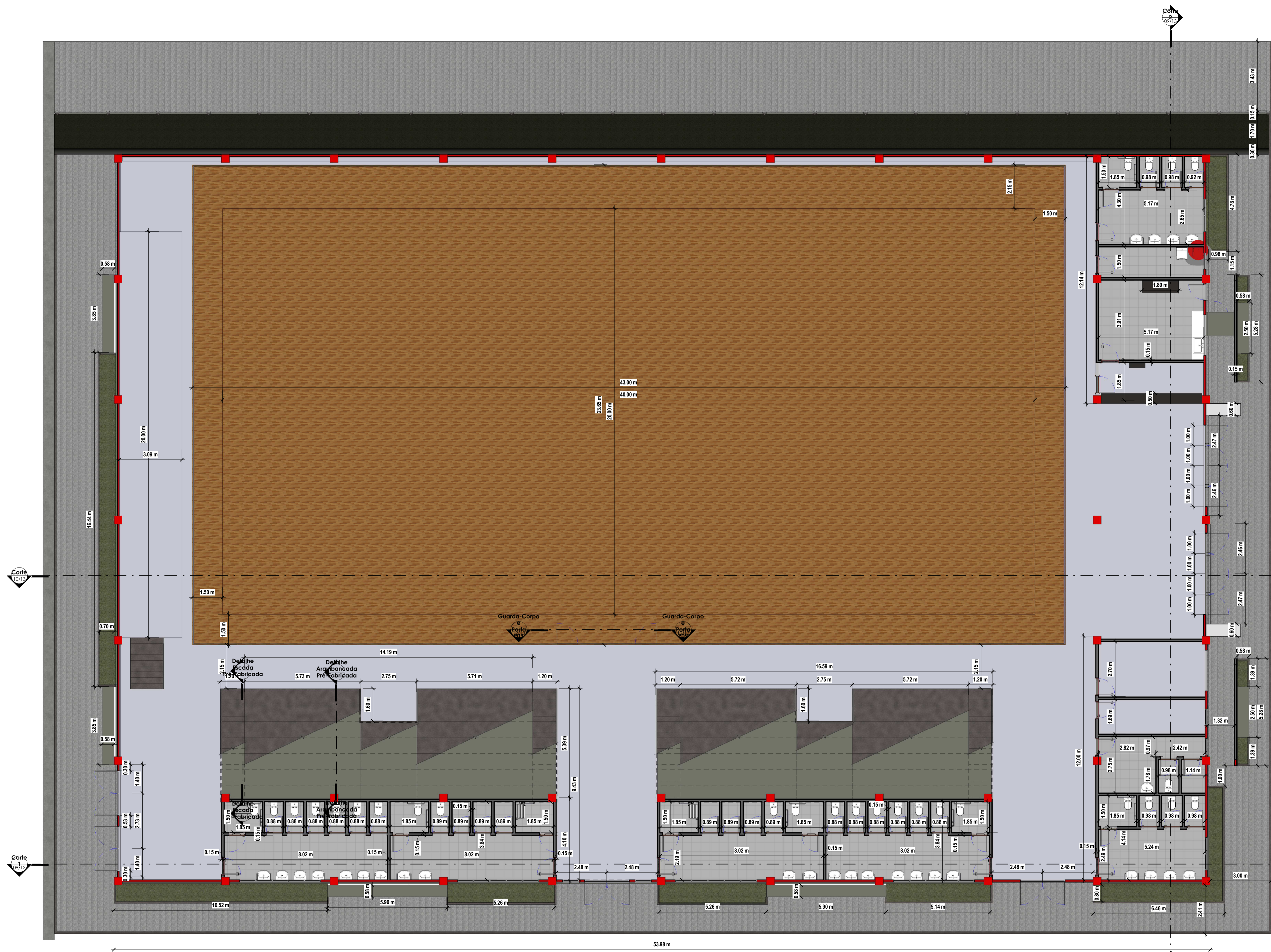
1 Planta de Térreo 1 : 100
