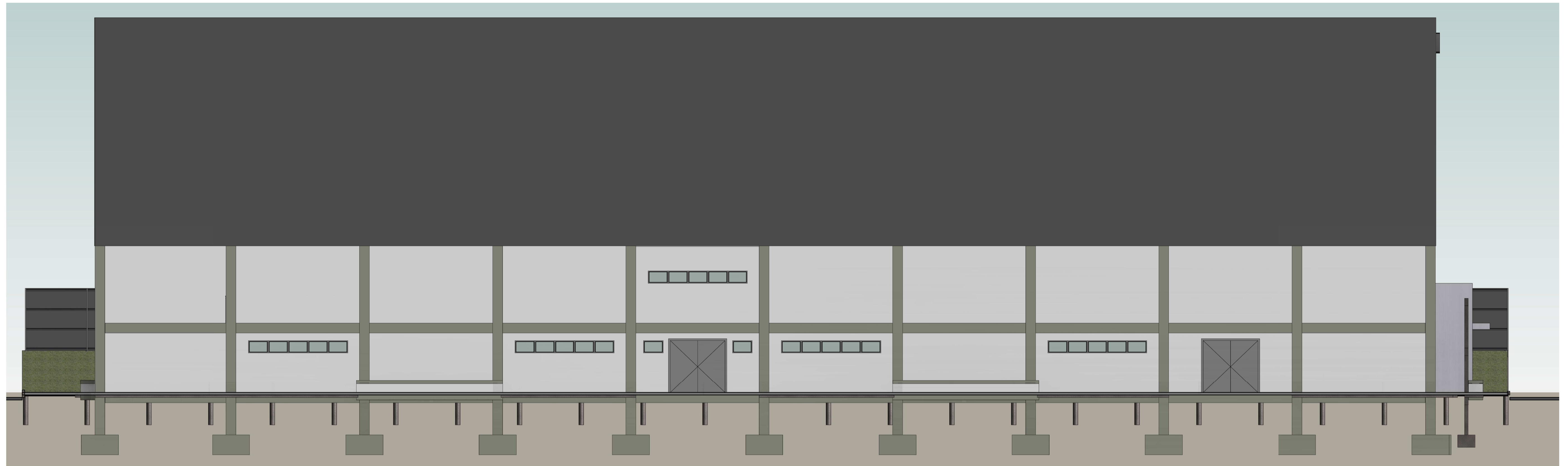
1 Fachada Lateral 1 : 85
