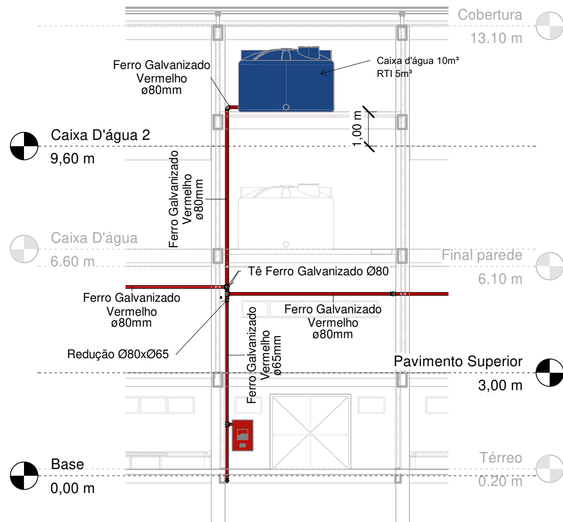
1 Detalhe Tubo Principal 1 : 100
