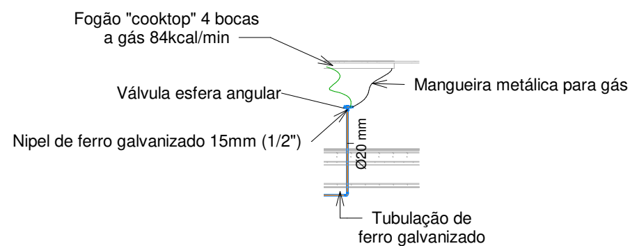
4 Corte 2 1 : 50
