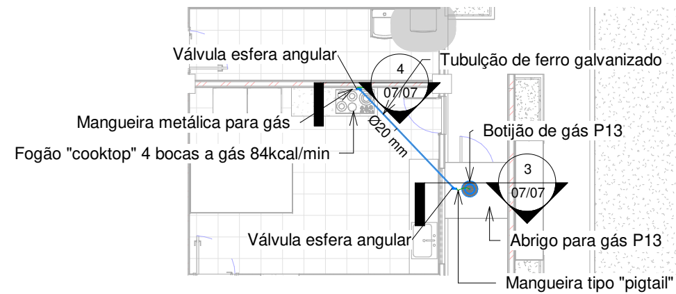
1 Planta Térreo 1 : 100
