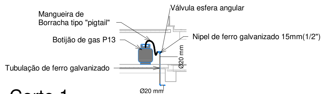
3 Corte 1 1 : 50
