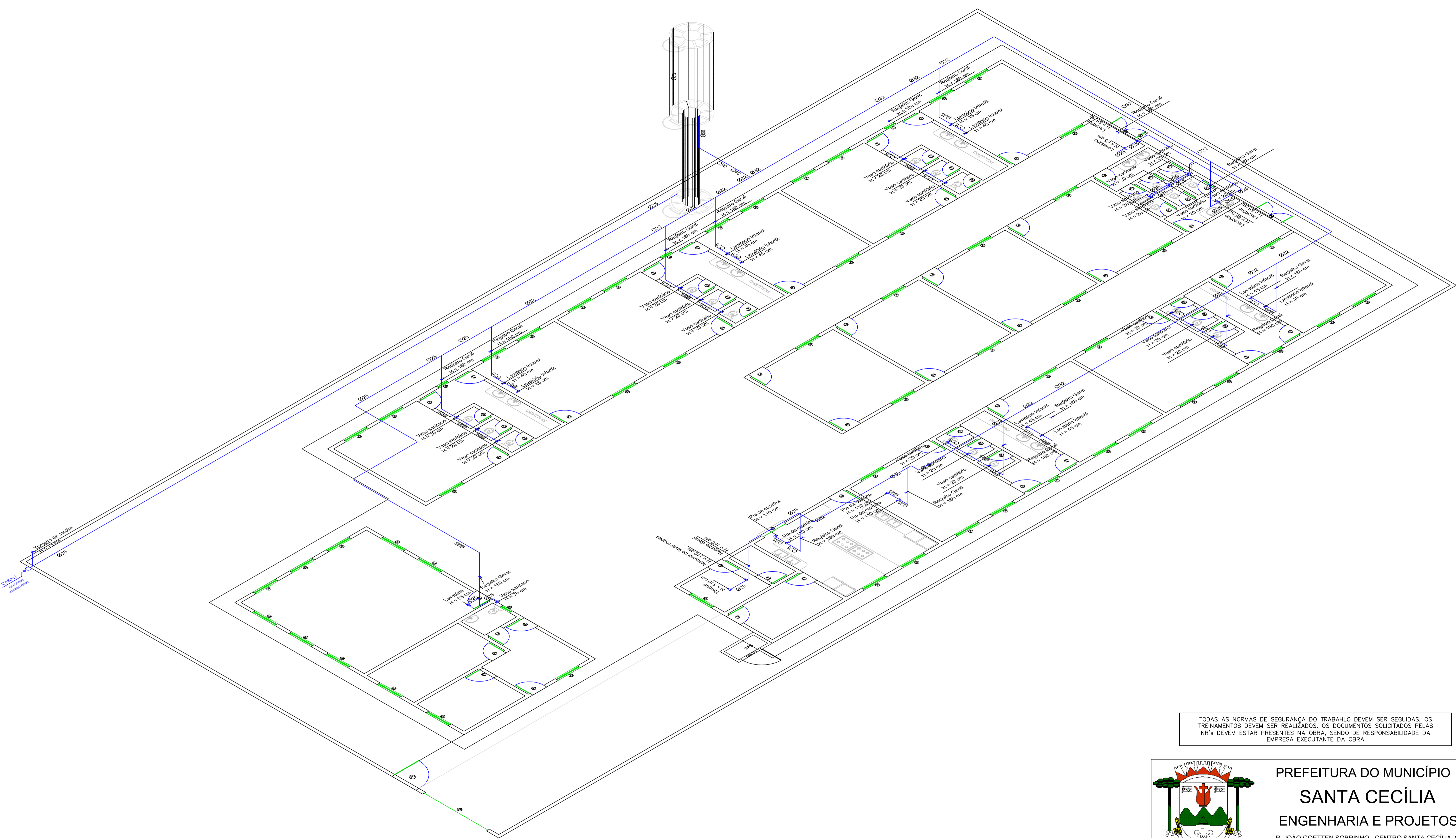
Isométrico Água Fria ESC.: 1:100
