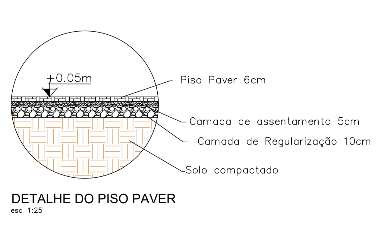
DETALHE DO PISO esc 1:25
