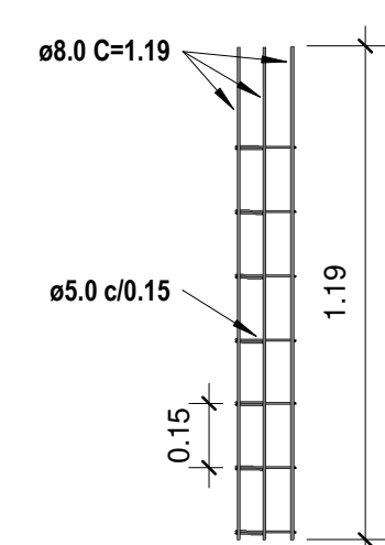
15 E1=E2=E3 1 : 20
