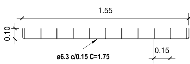
19 Armadura da Laje - Central GLP 02 1 : 20
