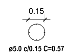
16 Estribos E1=E2=E3 1 : 20
