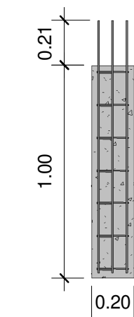
14 Concreto E1=E2=E3 1 : 25
