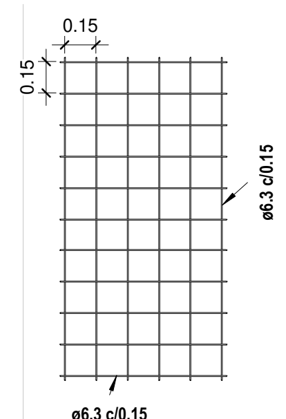
18 Armadura Laje - Central GLP 01 1 : 25
