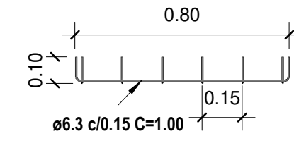
20 Armadura da Laje - Central GLP 03 1 : 20
