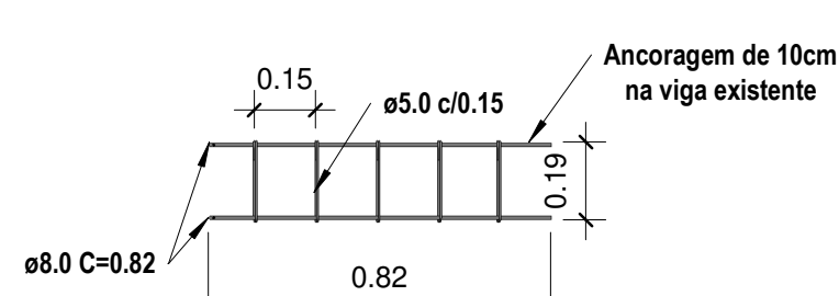
13 V6=V7 - Central GLP 1 : 20
