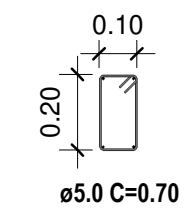
10 Estribos V5=V6=V7 - Central GLP 1 : 20
