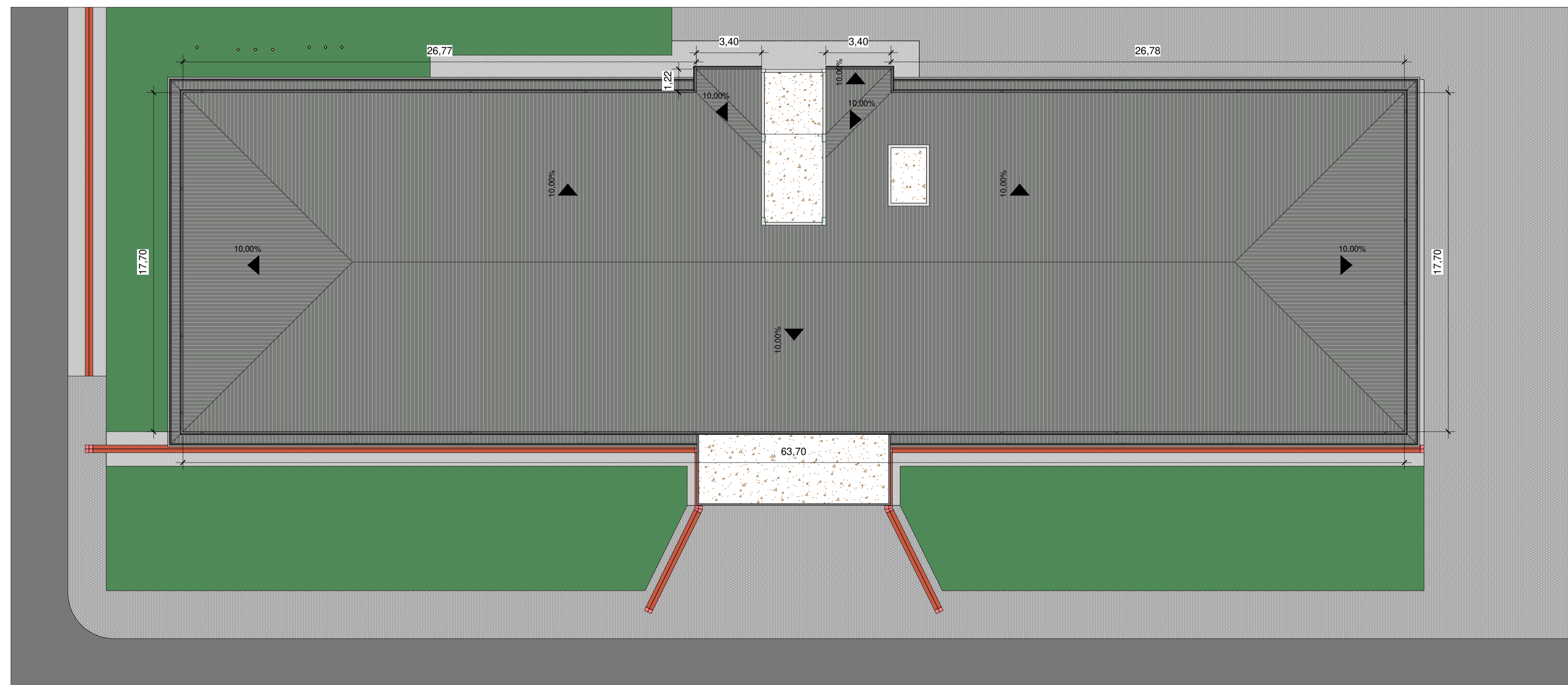
2 Cobertura Pav. Superior ESCALA 1 : 150
